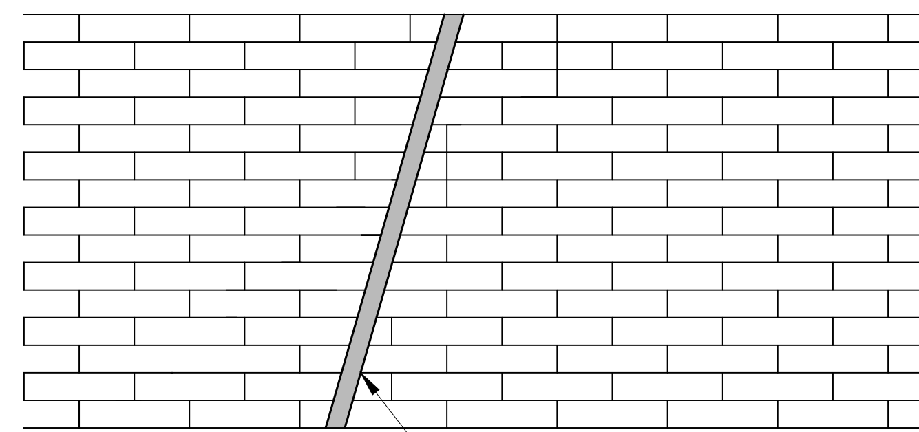
GRANITE ACCENT: 4'L x 4"W x 4"D
